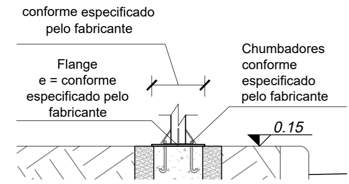
Espessura da flange poste 4m Esc.:1/20
