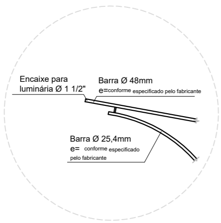
Detalhe Encaixe para luminária Ø 1 1/2" Esc.:1/50
