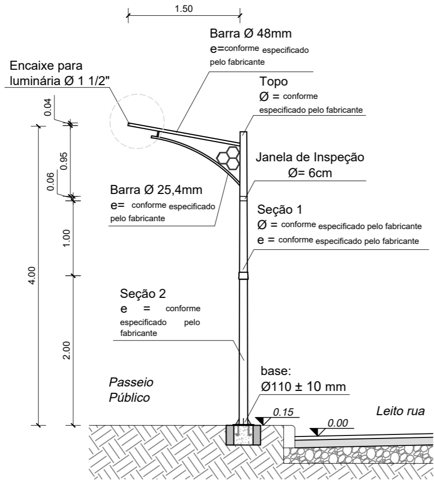
Poste Telefônico 4m - Modelo Pinhal - Braço Simples Esc.:1/50
