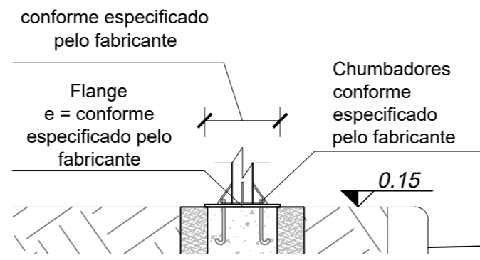
Espessura da flange poste 6m Esc.:1/20
