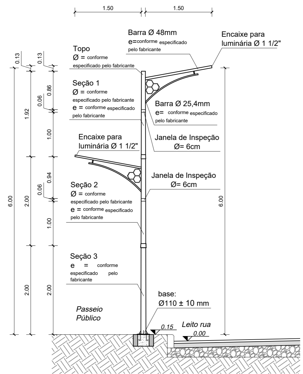
Poste Telefônico 6m - Modelo Pinhal - Braço Duplo Esc.:1/50
