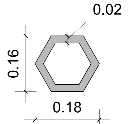
Favo de mel detalhe Esc.:1/5
