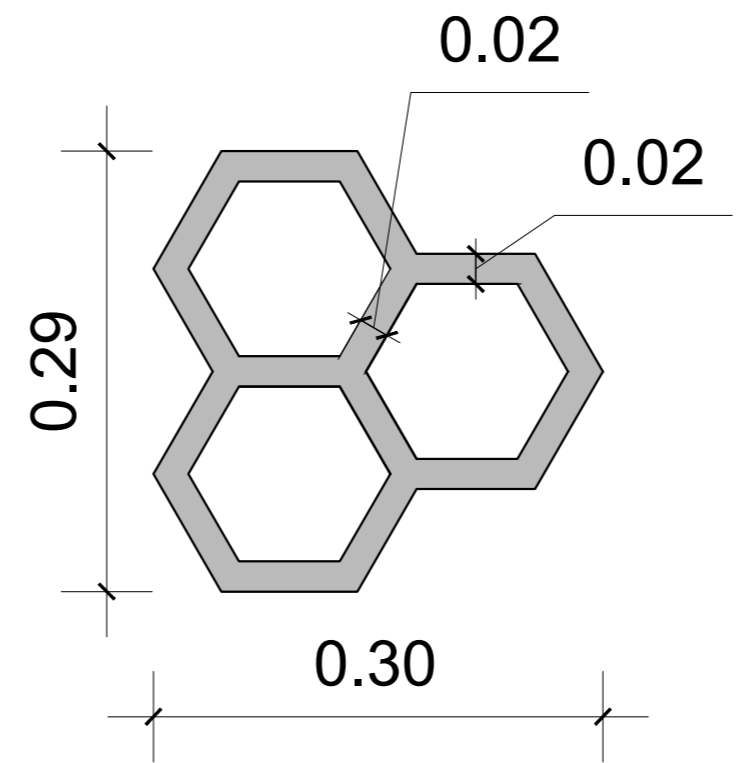
Favo de mel módulo Esc.:1/5
