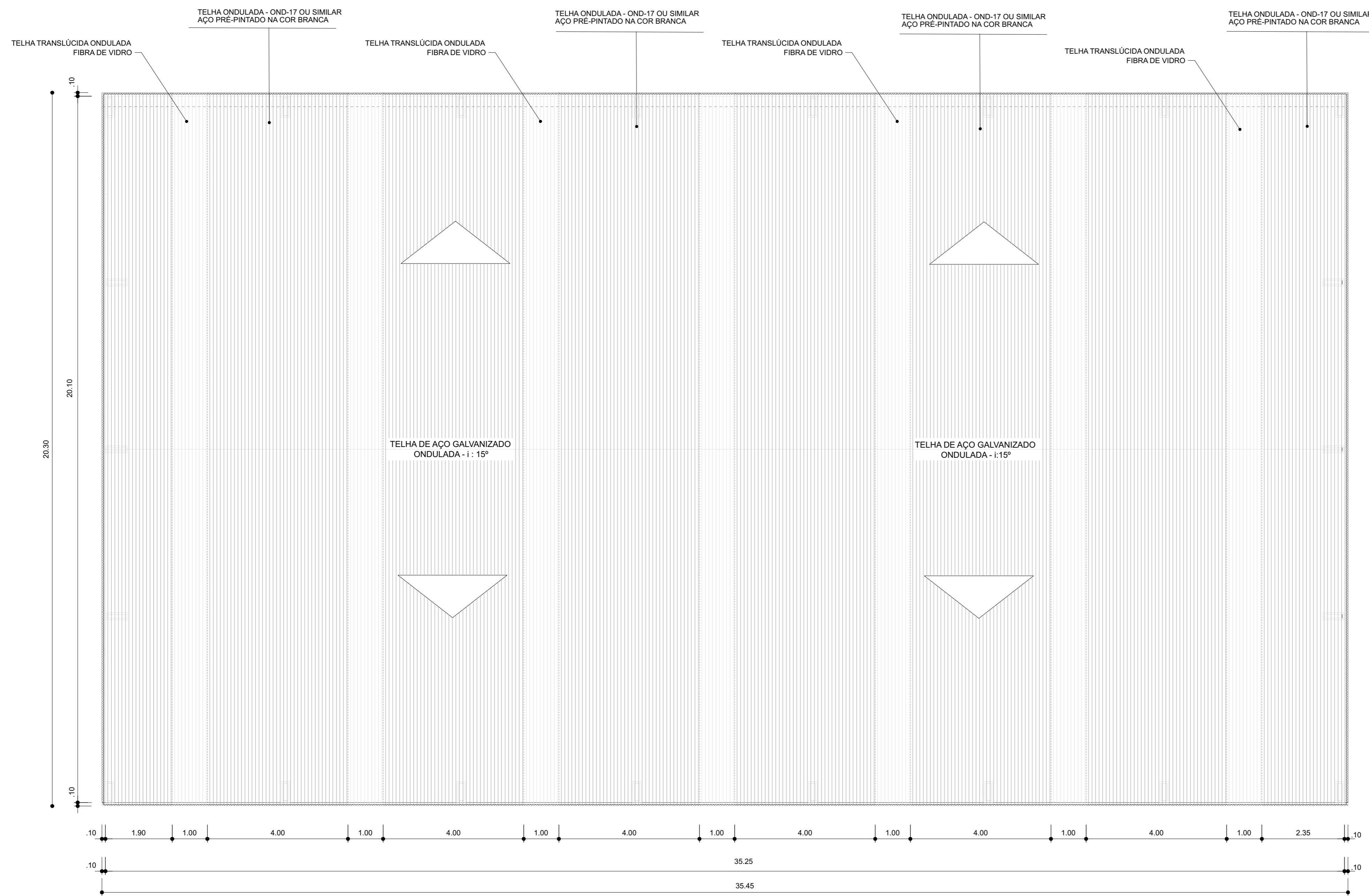
Planta de cobertura escala 1:75
