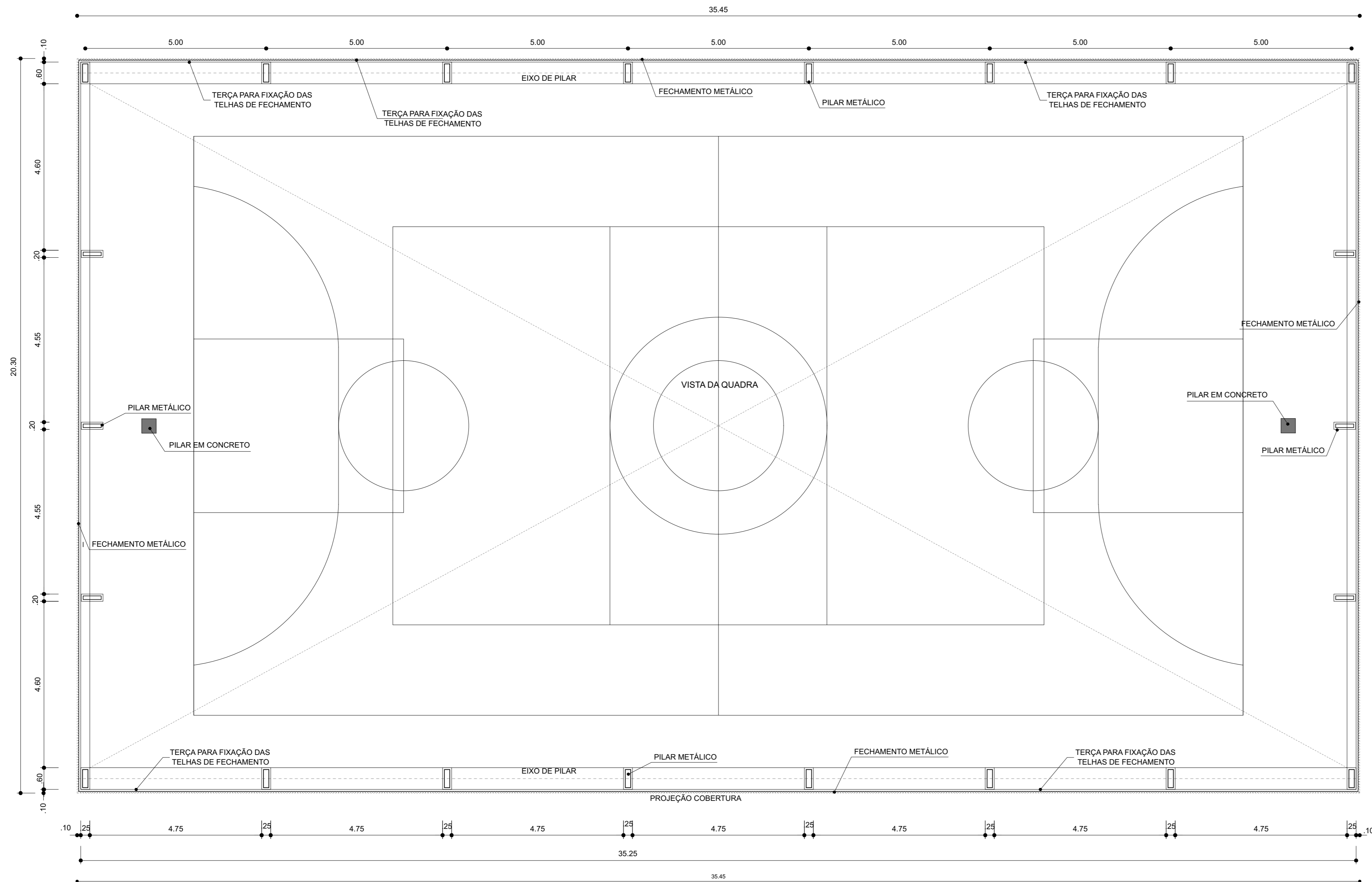
Planta baixa nivel fechamento escala 1:75
