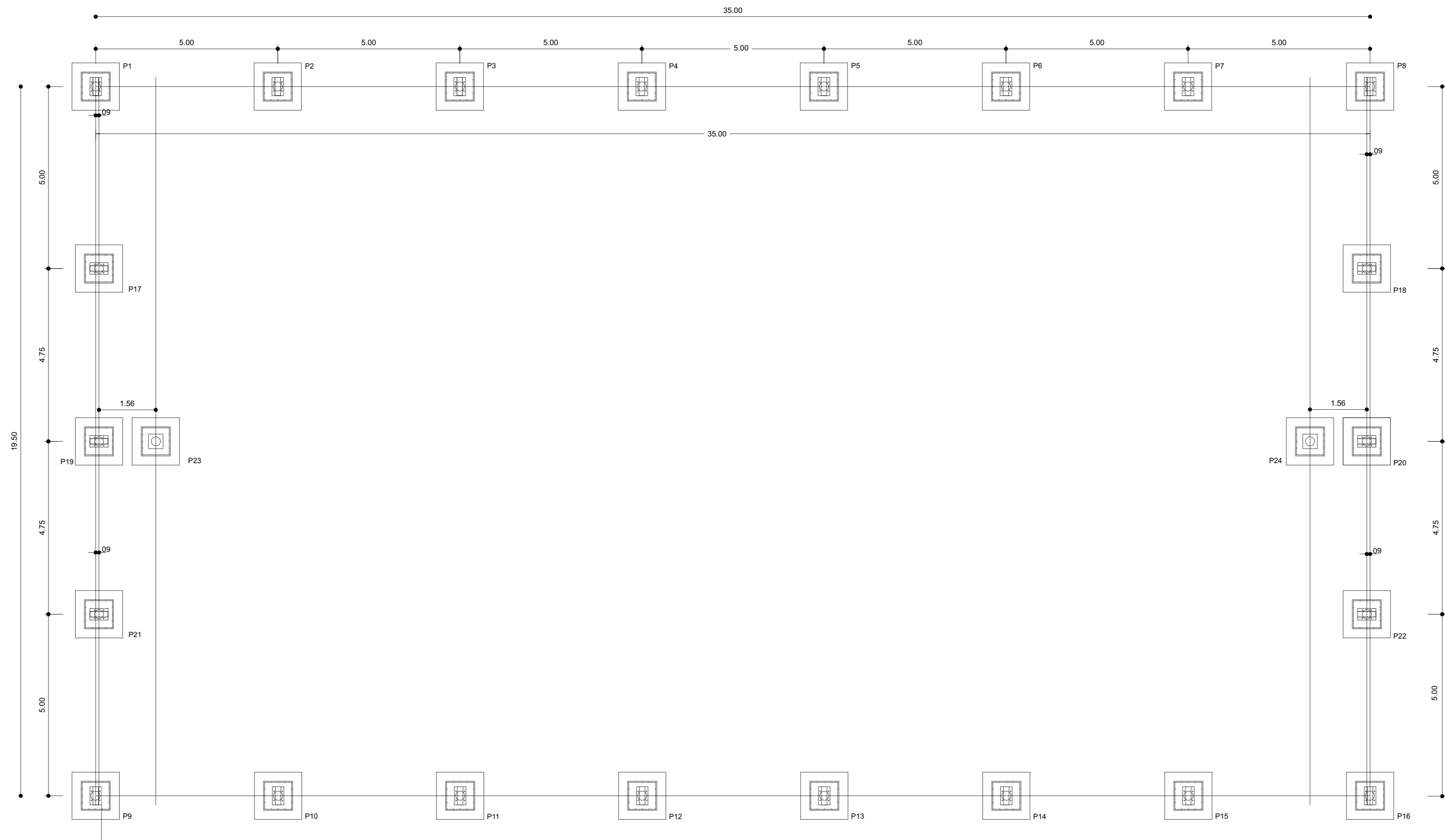
Planta dos blocos escala 1:75
