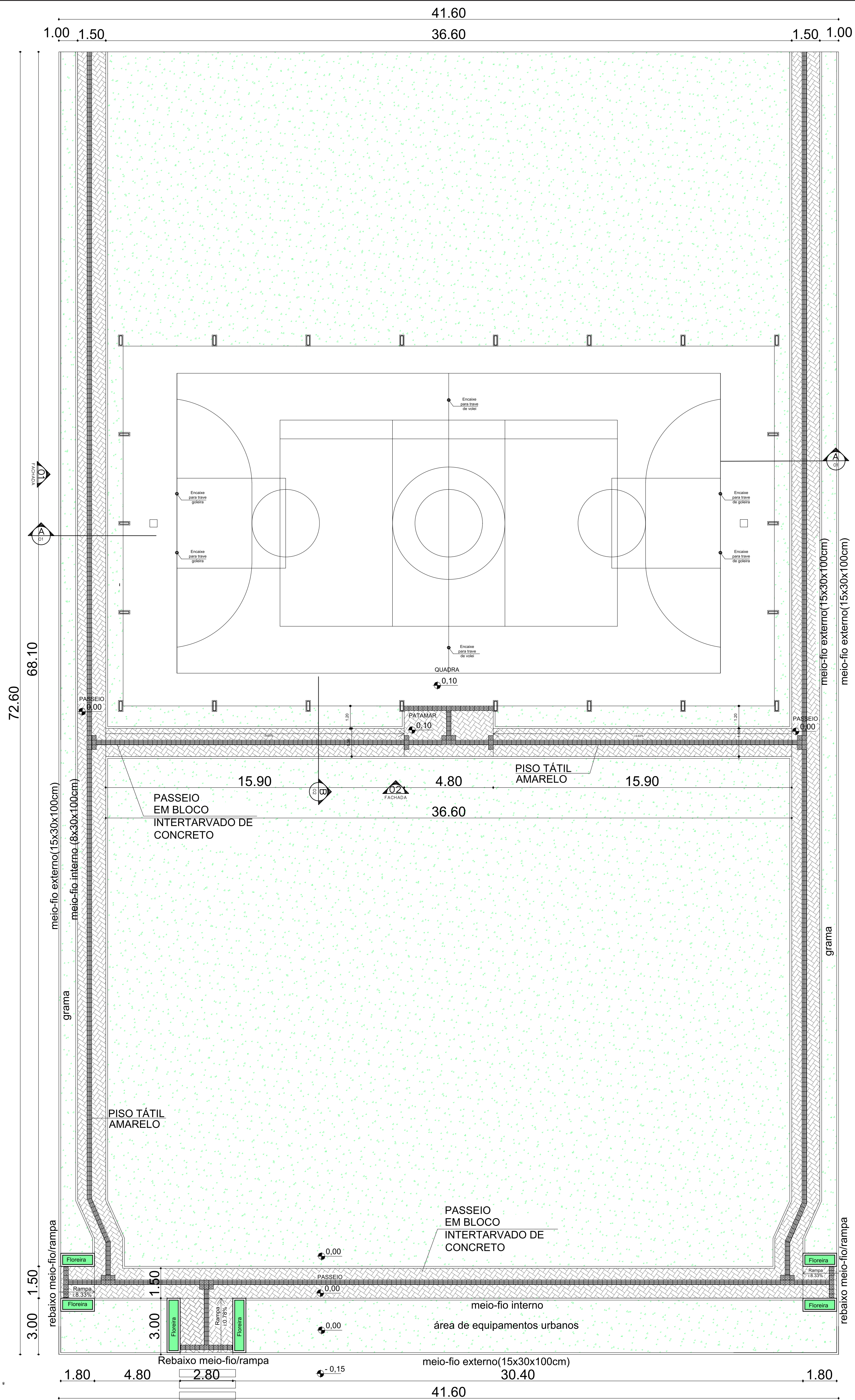
Planta de Acessibilidade escala 1:125
